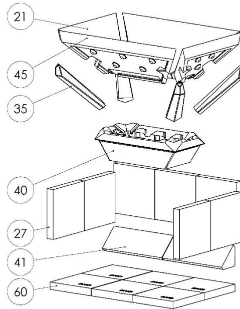
Anordnung der Formstücke nach Kesseltyp
