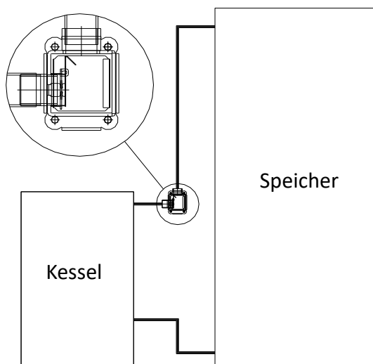
Anschluss am Vorlaufrohr vom Kessel
