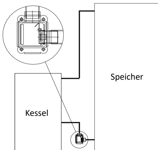
Anschluss am Rücklaufrohr zum Kessel
