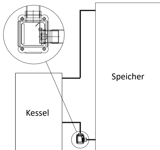
Anschluss am Rücklaufrohr zum Kessel
