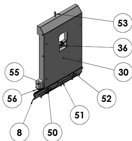
Detal A – kolektor powietrza
