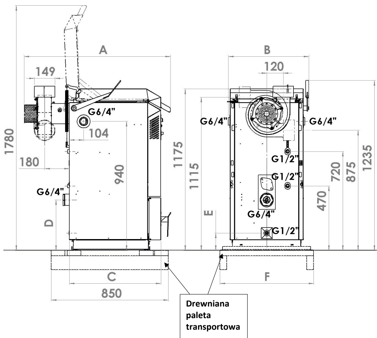
Wymiary korpusu kotła.
