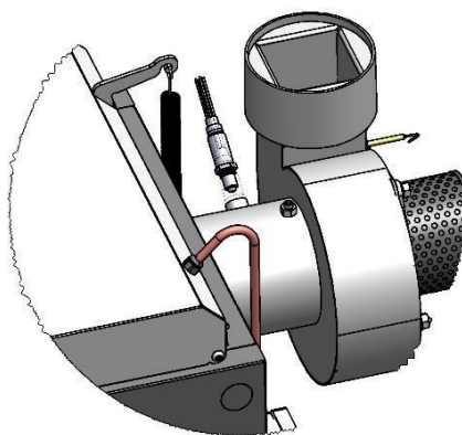
Instalacja sondy lambda na czopuchu kotła
