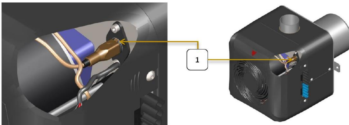
Rysunek 29. Czyszczenie czujnika optycznego
