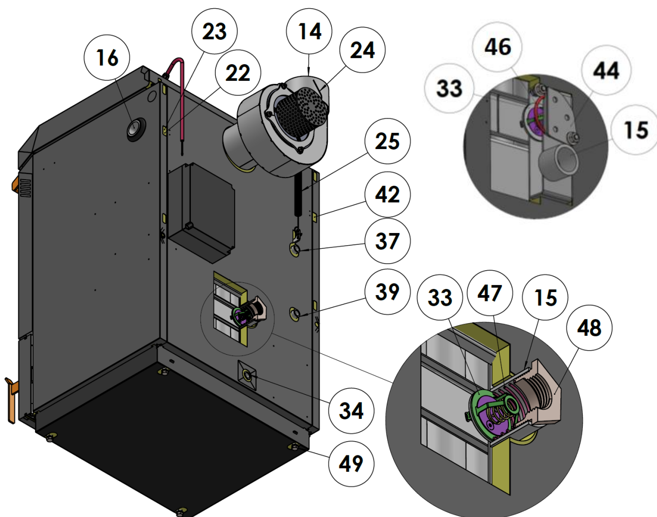
Schema della caldaia - vista posteriore (senza ESP)
