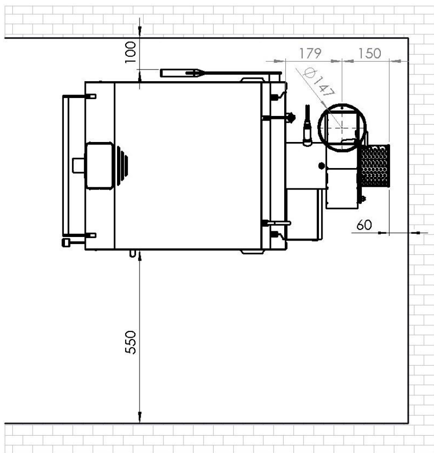
Dimensioni minime per la collocazione della caldaia (senza ESP)
