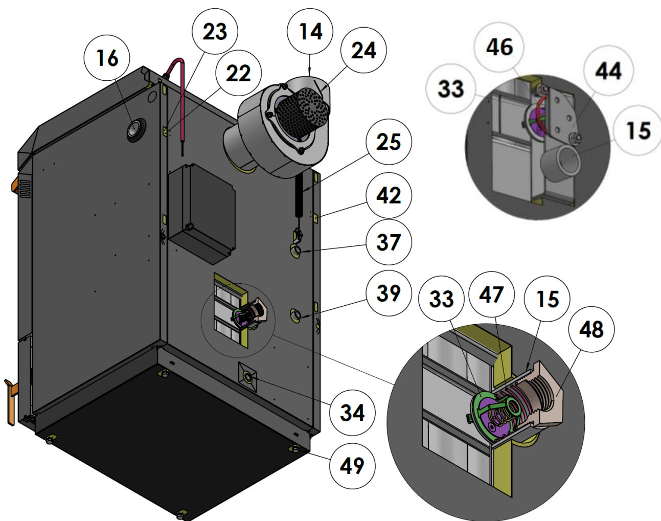
Schema della caldaia - vista posteriore
