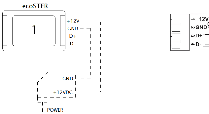
Obrázek 25. Dvouvodičové připojení pokojového panelu ecoSTER
