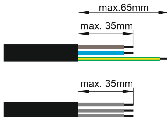
Obrázek 11. Délka odizolování kabelů
