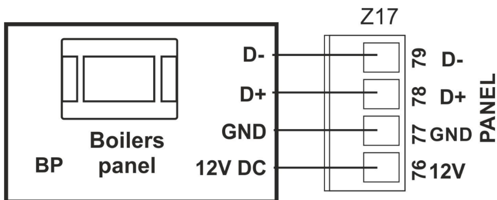
Obrázek 13. Elektrické schéma zapojení ovládacího panelu regulátoru
