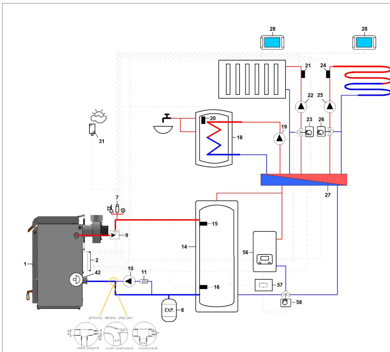
Obrázek 29. Hydraulické zapojení s rezervním kotlem (56), relé (57) a přepínacím ventilem (58)
