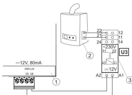
Obrázek 27. Elektrické připojení rezervního kotle:
