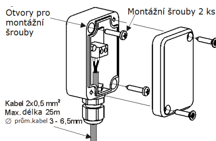
Obrázek 19. Připojení čidla venkovní teploty CT10P (není v základní výbavě kotle)
