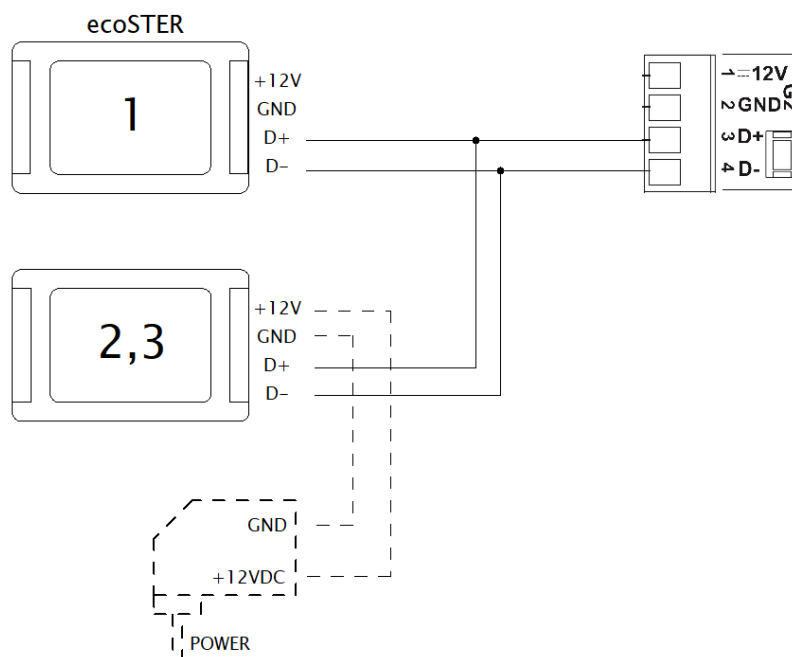
Obrázek 26. Kombinované připojení pokojového panelu ecoSTER
