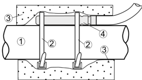
Obrázek 17. Instalace teplotního čidla na trubku,
