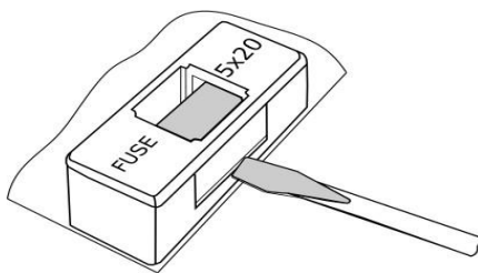
Obrázek 9. Výměna síťové pojistky
