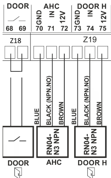
Obrázek 16. Elektrické schéma zapojení indukčních čidel
