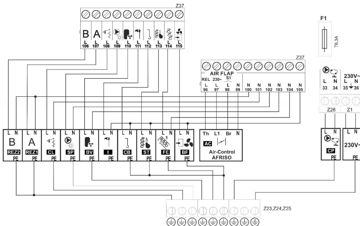
Obrázek 31. Připojení ostatních periférií 1
