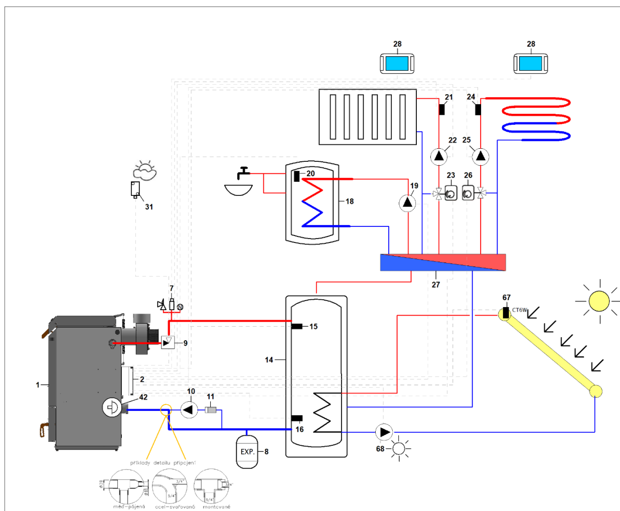
Obrázek 8. Hydraulické zapojení se solárním kolektorem:
