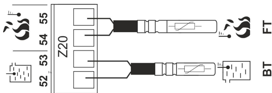
Obrázek 18. Připojení teplotních čidel,
