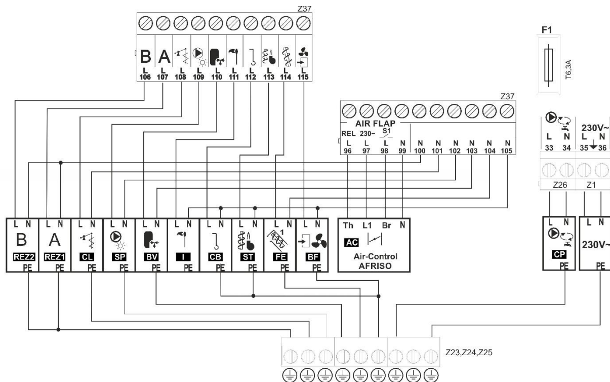
Obrázek 36: Připojení ostatních periférií 1
