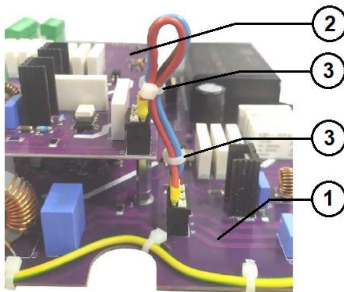
Obrázek 16: Propojení modulu P s modulem A
