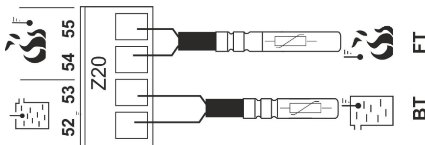
Obrázek 23: Připojení teplotních čidel
