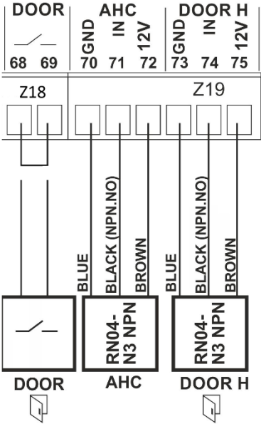
Obrázek 20: Elektrické schéma zapojení indukčních čidel
