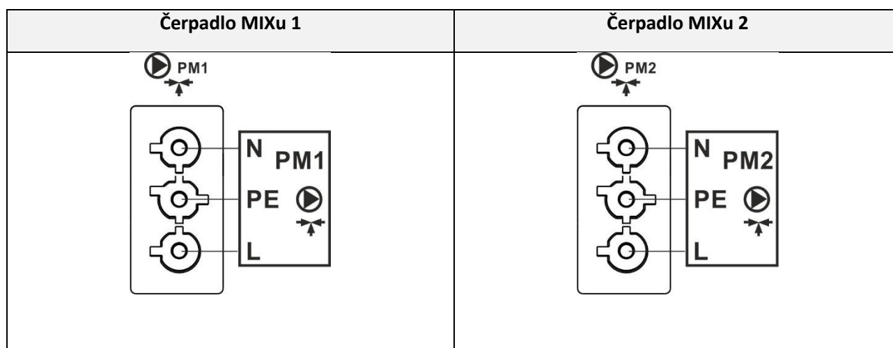
Obrázek 27: Elektrické schéma zapojení čerpadel MIXů
