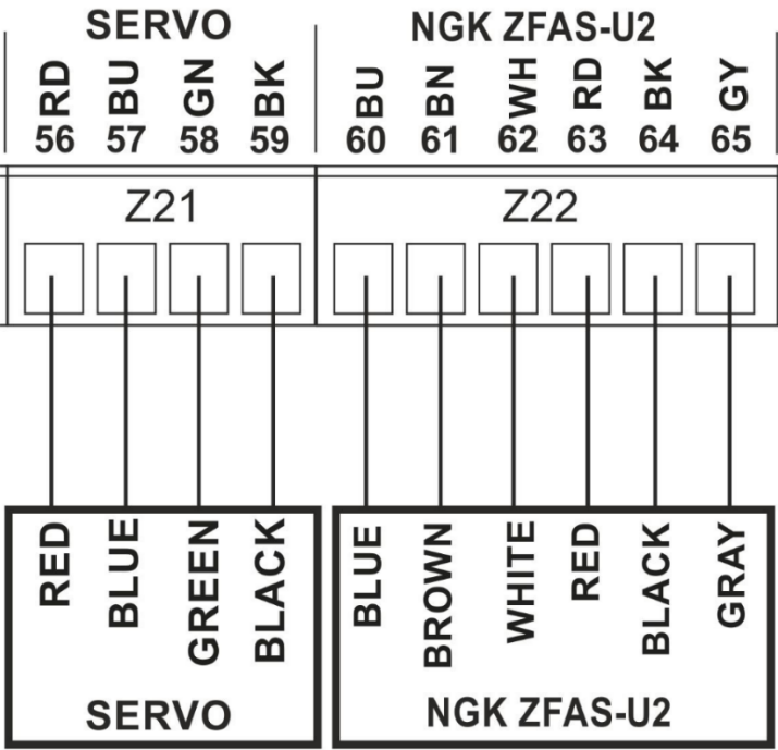
Obrázek 19: Elektrické schéma zapojení lambda sondy (NGK ZFAS-U2) a krokového motoru (SERVO)
