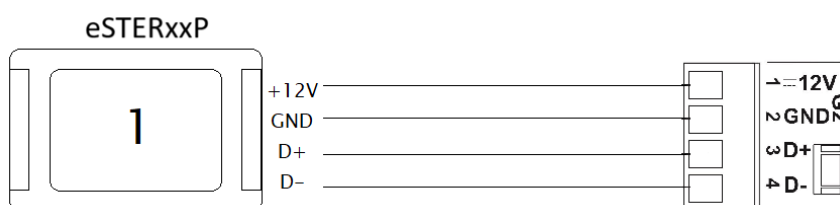
Obrázek 29: Čtyřvodičové připojení pokojového panelu eSTERxxP
