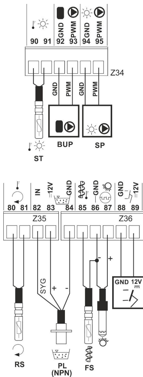
Obrázek 37: Připojení ostatních periférií 2
