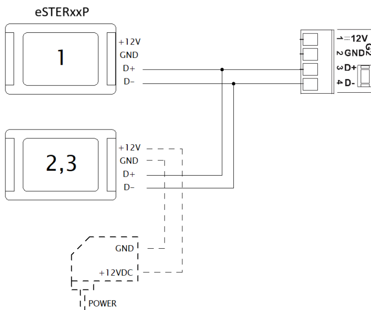
Obrázek 31: Kombinované připojení pokojového panelu eSTERxxP
