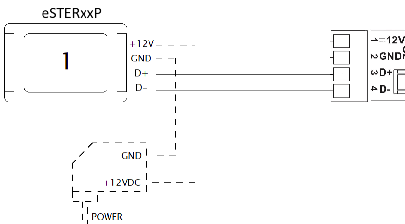
Obrázek 30: Dvouvodičové připojení pokojového panelu eSTERxxP
