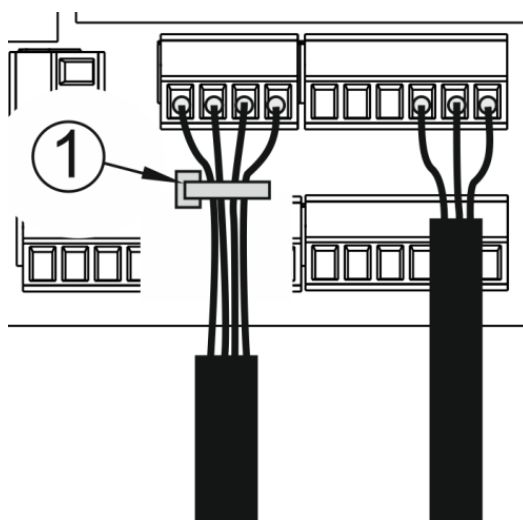
Obrázek 15: Délka odizolování kabelů
