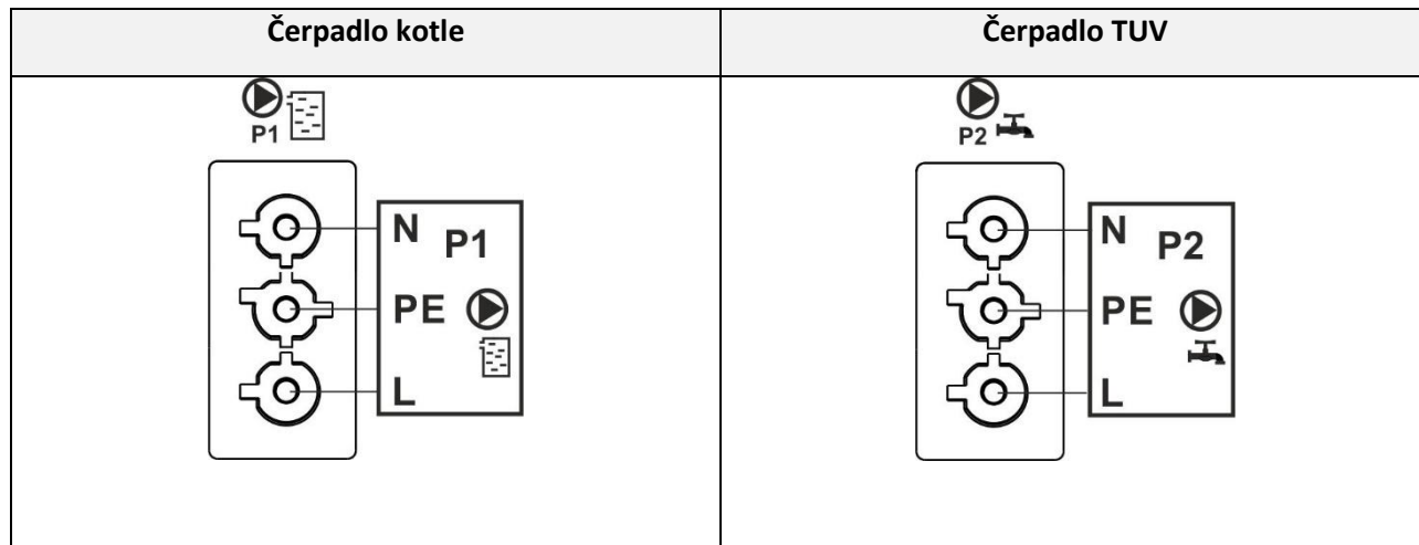
Obrázek 26: Elektrické schéma zapojení čerpadla kotle a čerpadla TUV
