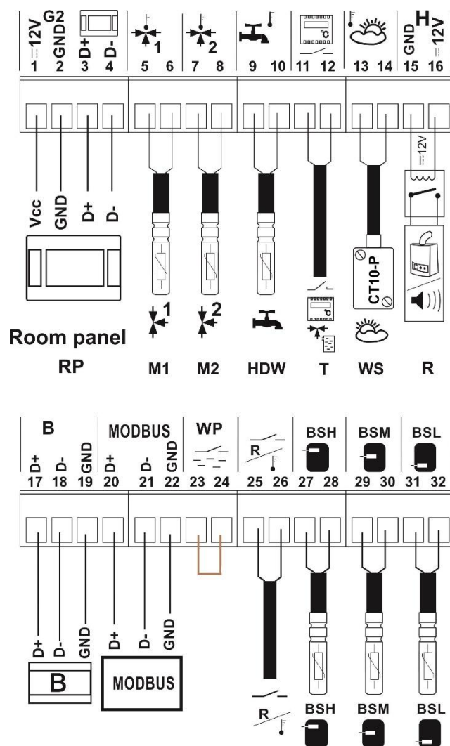
Obrázek 25: Elektrické schéma zapojení čidel a pokojového panelu
