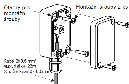
Obrázek 24: Připojení čidla venkovní teploty CT10P
