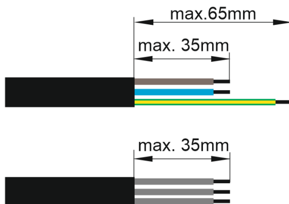
Obrázek 14: Délka odizolování kabelů
