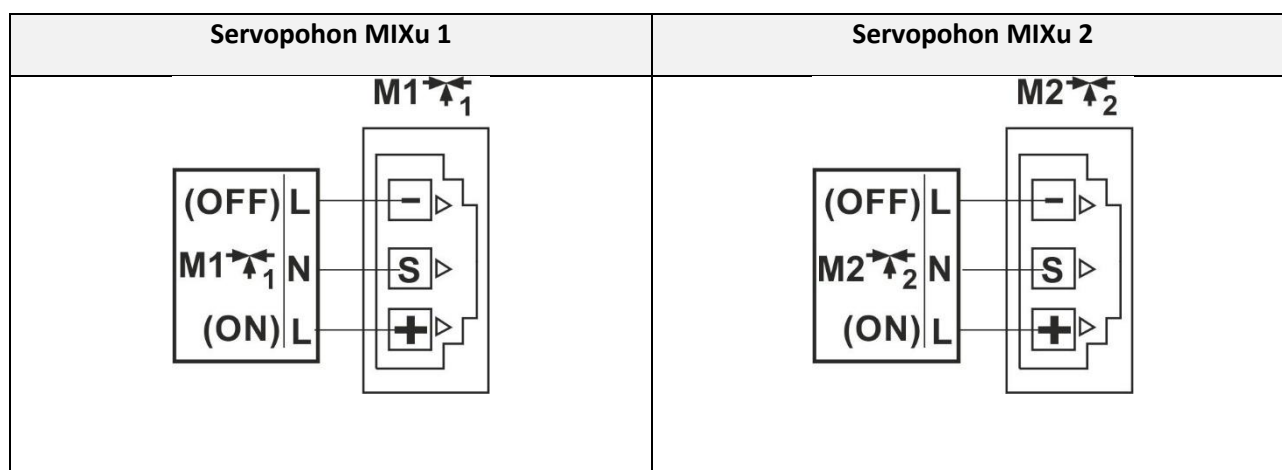
Obrázek 28: Elektrické schéma zapojení servopohonů MIXů
