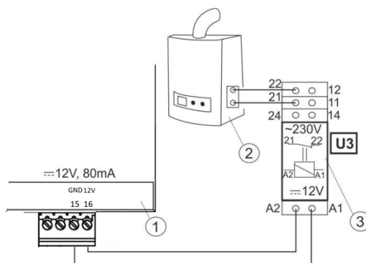
Obrázek 32: Elektrické připojení rezervního kotle
