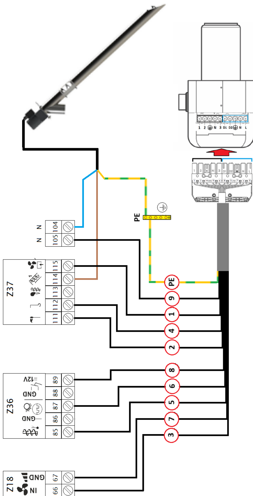
Elektrické schéma zapojení signálního kabelu hořáku a podavače
