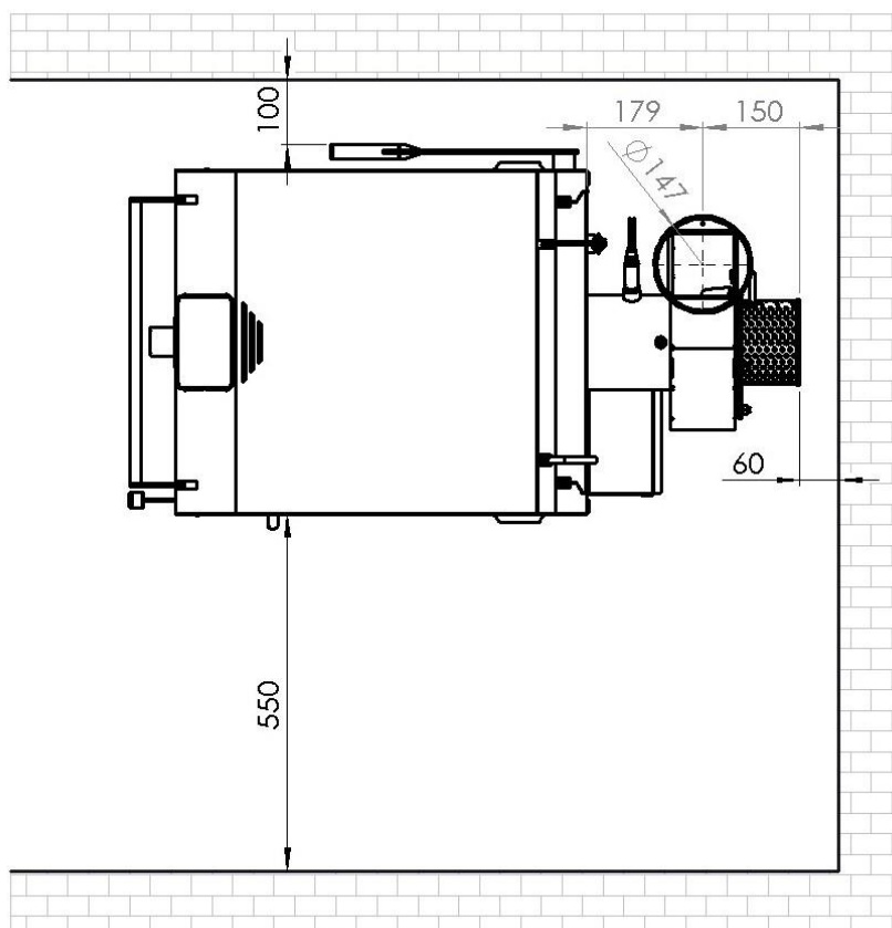
Minimálne rozmery pre umiestnenie kotla
