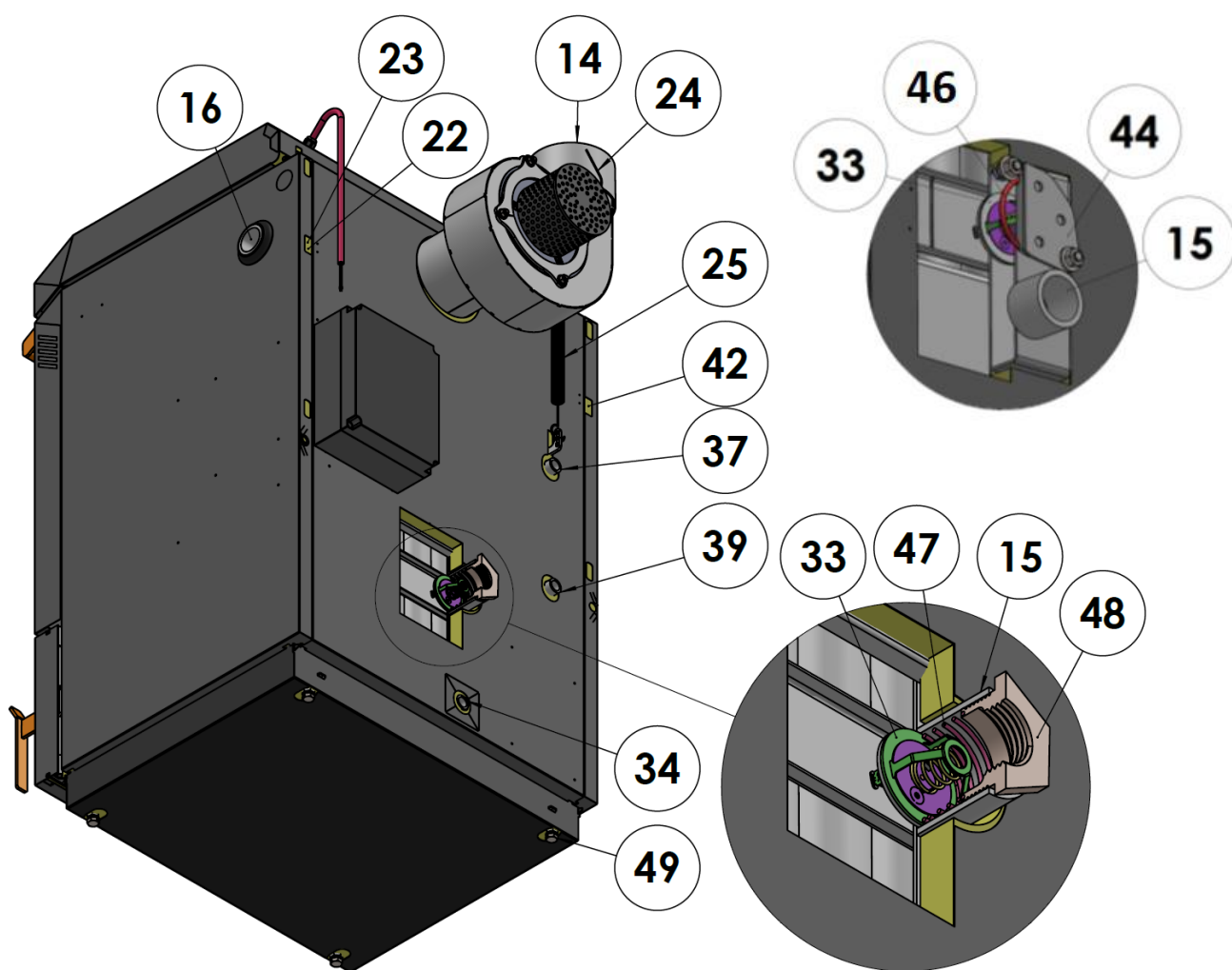
Schéma kotla – pohľad zozadu
