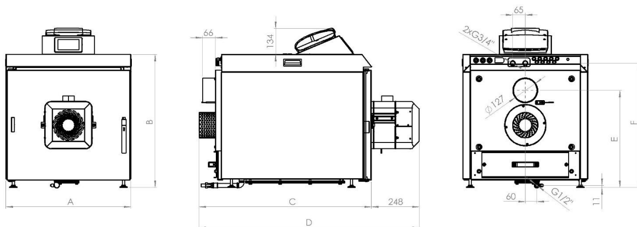
Tabulka základních rozměrů kotle bez zásobníku, bez odpopelňovače
