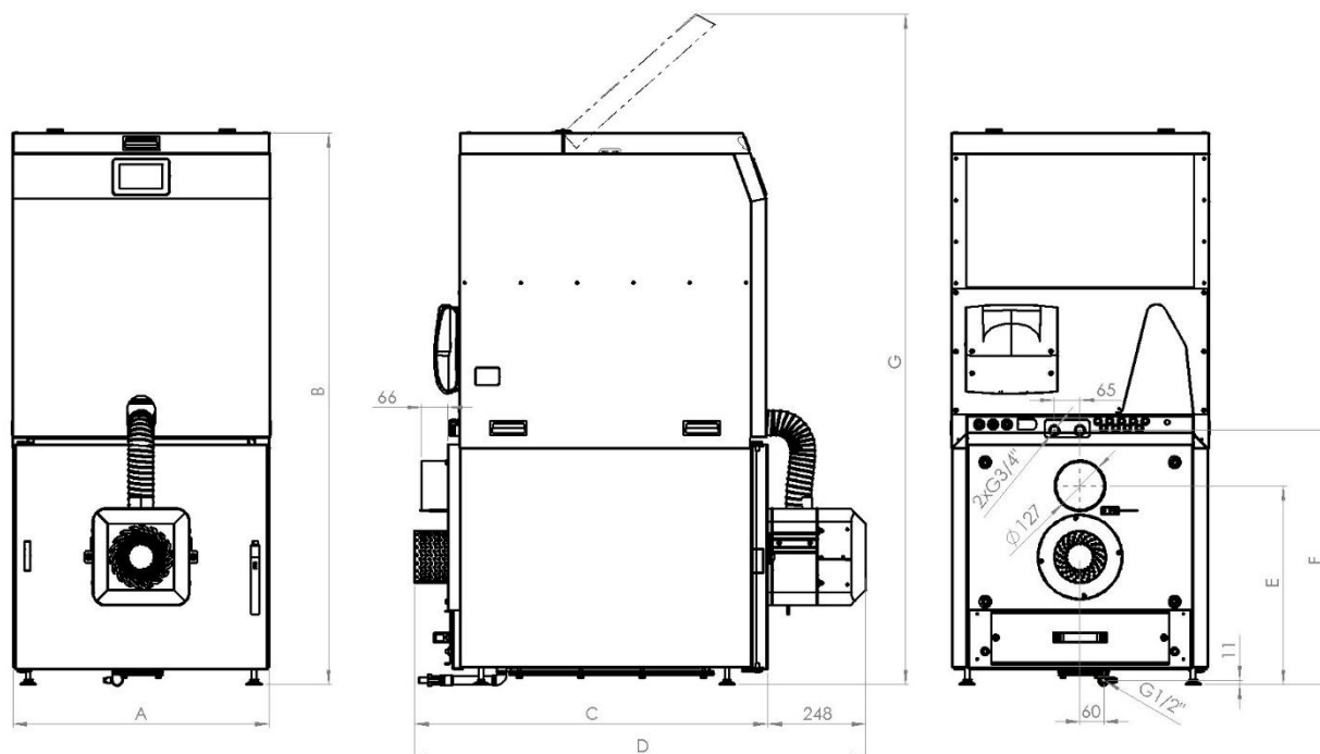
Tabulka základních rozměrů kotle s integrovaným zásobníkem, bez odpelňovače
