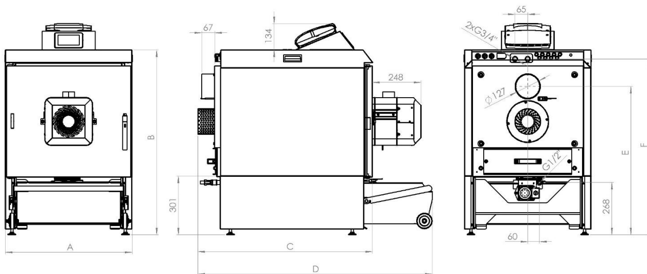
Tabulka základních rozměrů kotle bez zásobníku, s odpelňovačem
