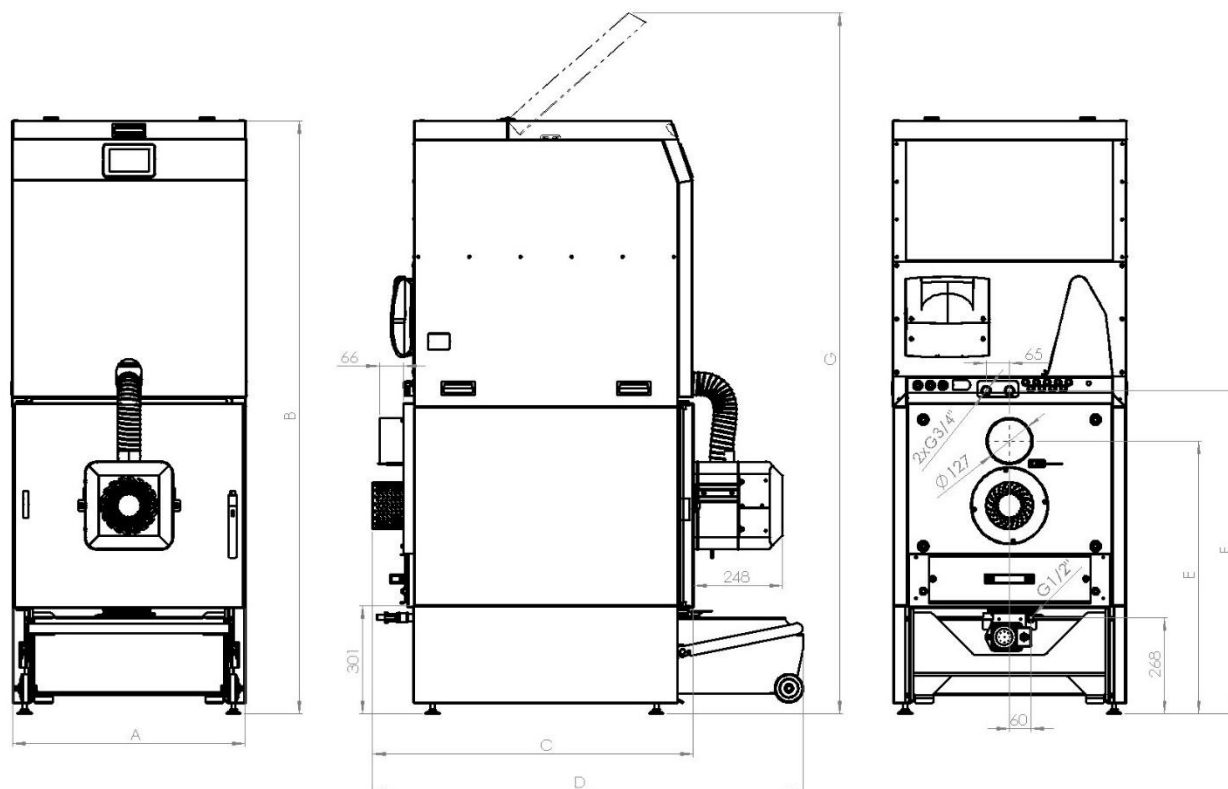
Tabulka základních rozměrů kotle s integrovaným zásobníkem, s odpelňovačem
