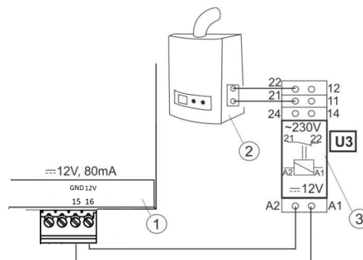
Abbildung 26: Elektrischer Anschluss des Reservekessels:
