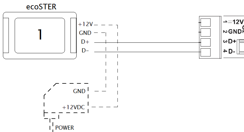
Abbildung 24: Zweidrahtanschluss des ecoSTER-Raumbediengerätes
