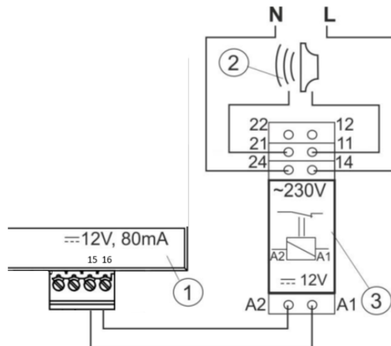
Abbildung 29. Anschluss eines externen Geräts zur Signalisierung eines Alarms, wobei: 1 - Regler, 2 - externer Alarmgeber, 3 - Relais
