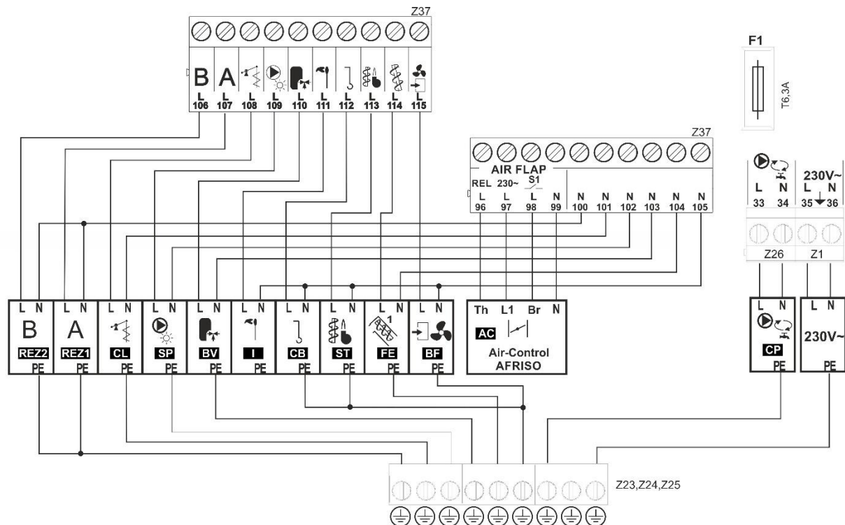
Abbildung 30. Anschließen anderer Peripheriegeräte 1
