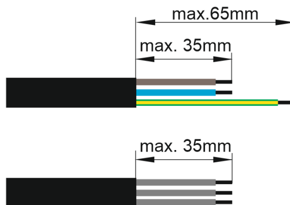
Abbildung 10. Abisolierlänge des Kabels
