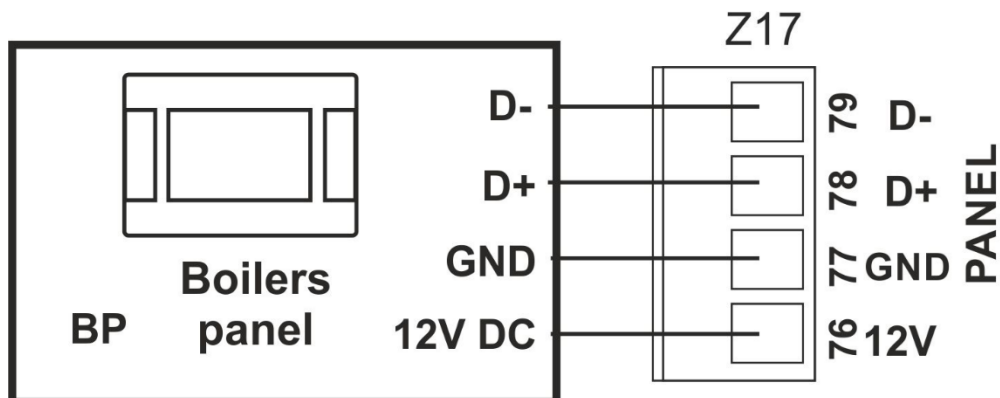
Abbildung 12: Schaltplan für das Steuerpult des Reglers
