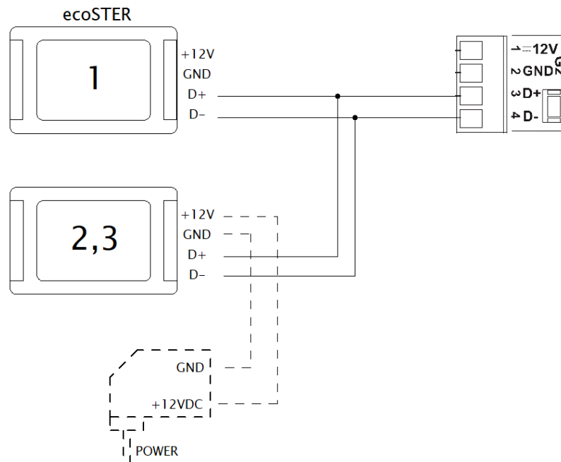
Abbildung 25: Anschluss des kombinierten ecoSTER-Raumbediengerätes
