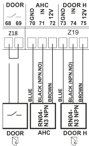
Abbildung 15: Anschlussplan für induktive Sensoren
