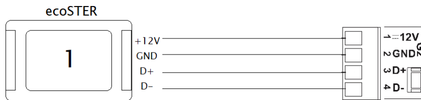
Abbildung 23: Vierdrahtanschluss des ecoSTER-Raumbediengerätes
