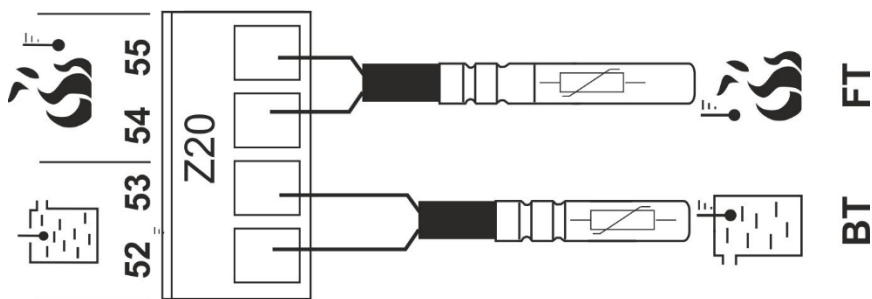
Abbildung 17: Anschluss der Temperatursensoren,
