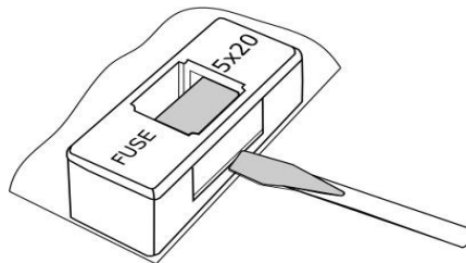
Abbildung 8: Auswechseln der Netzsicherung
