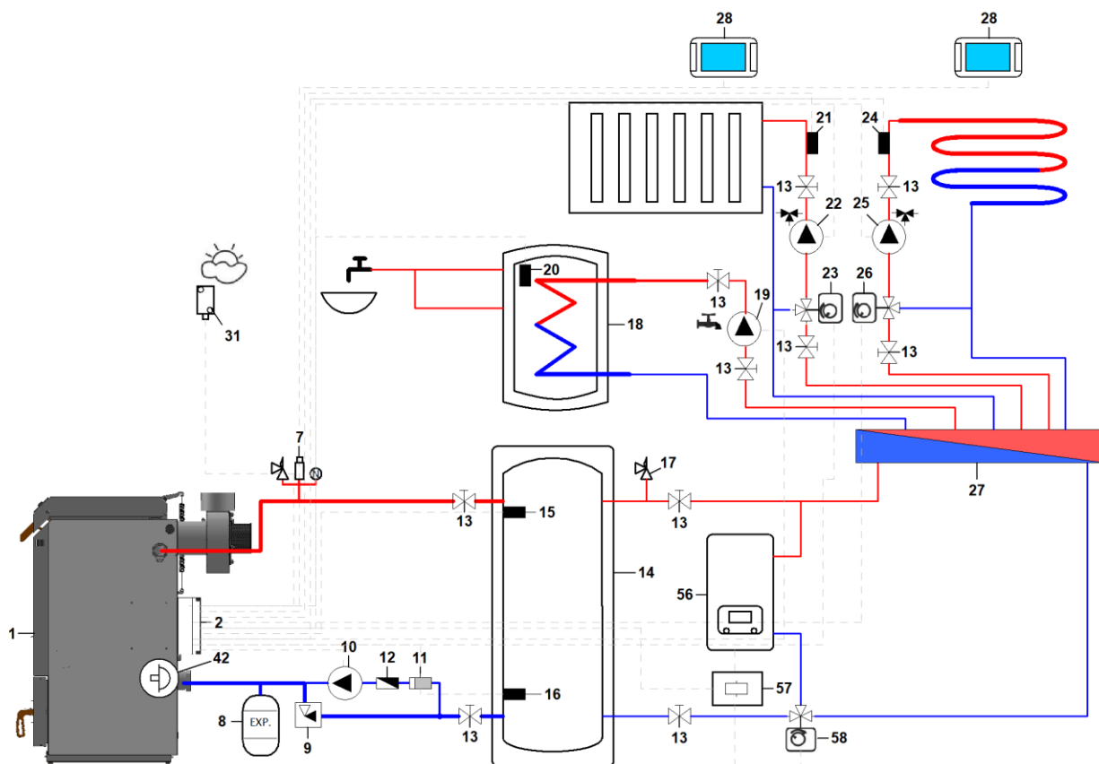
Abbildung 28. Hydraulischer Anschluss mit Reservekessel (56) und Umlenkventil (58)
