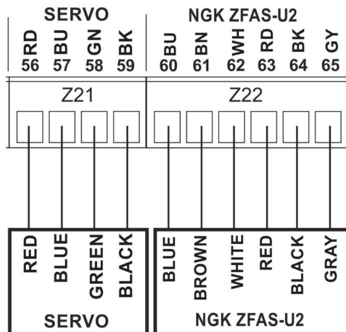
Abbildung 14: Schaltplan für Lambdasonde (NGK ZFAS-U2) und Schrittmotor (SERVO)
