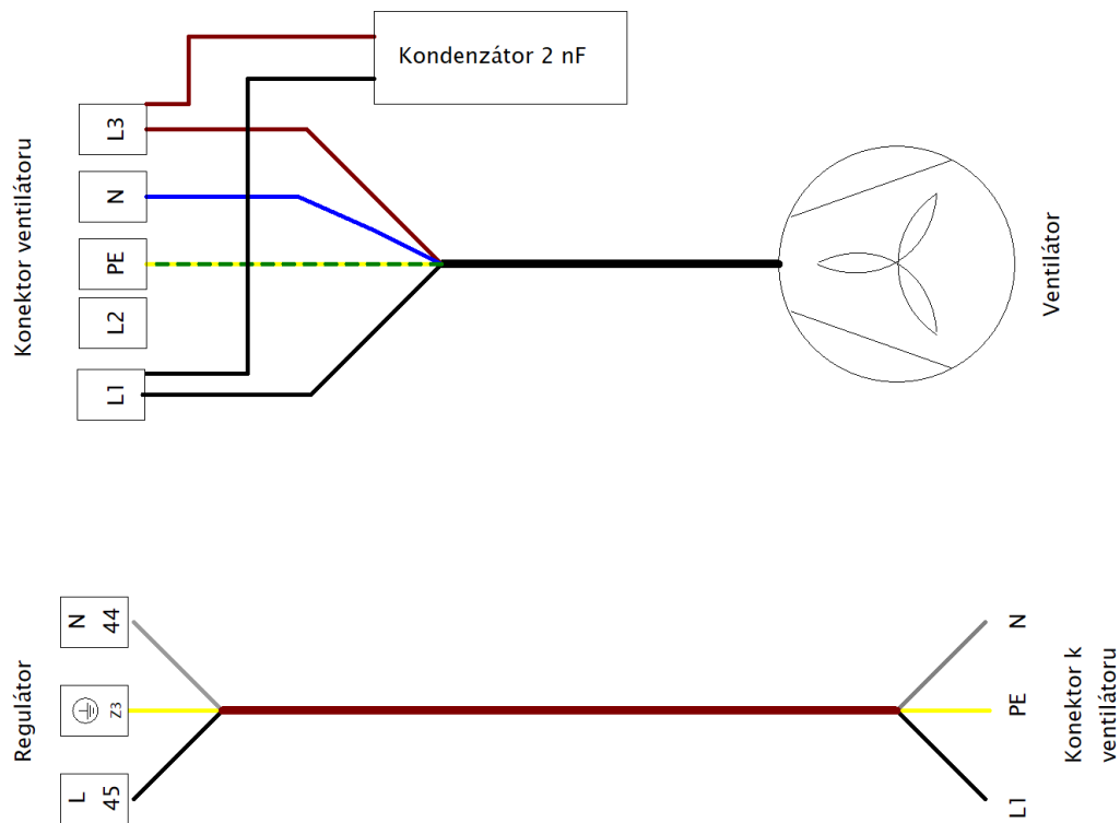
Abbildung 13: Elektrischer Schaltplan für den Abluftventilator
