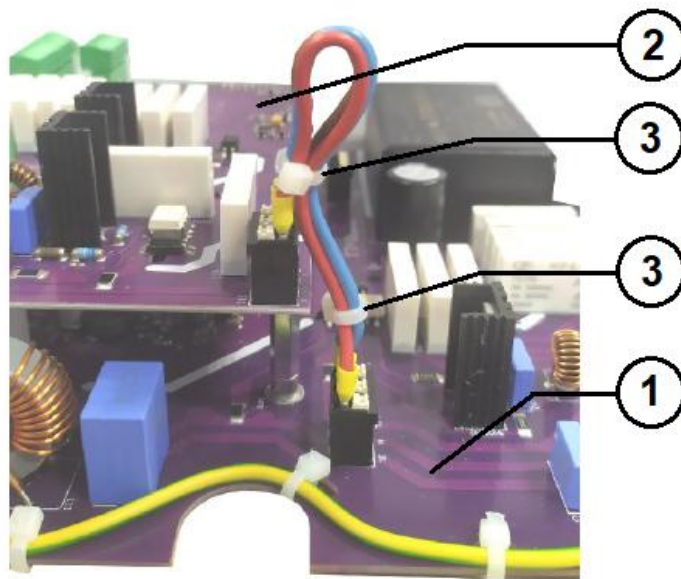
Rysunek 14. Łączenie modułu P z modułem A, gdzie: 1 – płyta modułu A, 2 – płyta modułu P, 3 – opaska kablowa
