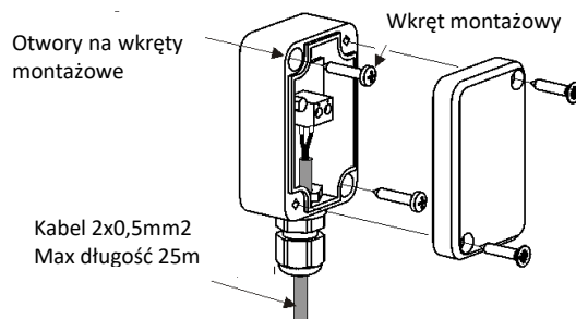
Rysunek 22. Podłączenie czujnika temperatury zewnętrznej CT10P (brak w podstawowym wyposażeniu kotła)
