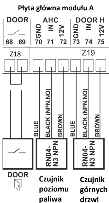
Rysunek 18. Schemat elektryczny czujników indukcyjnych
