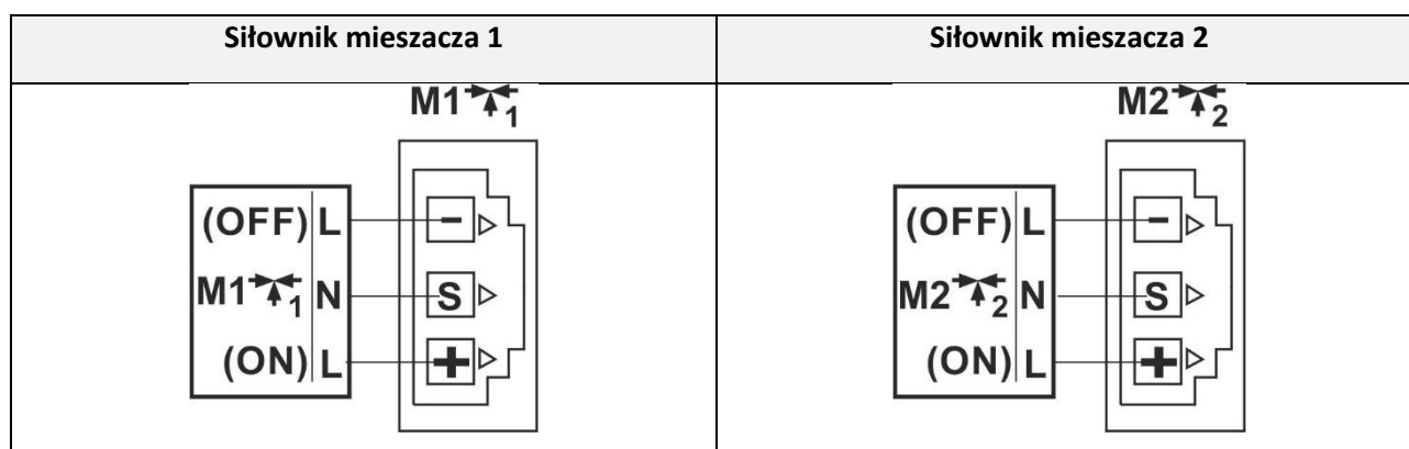
Rysunek 26. Schemat elektryczny siłowników mieszaczy
