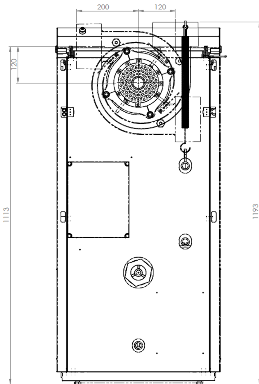
Zadní pohled na kotel BLAZE PRAKTIK COMBI 25 a 40 s rozměry
