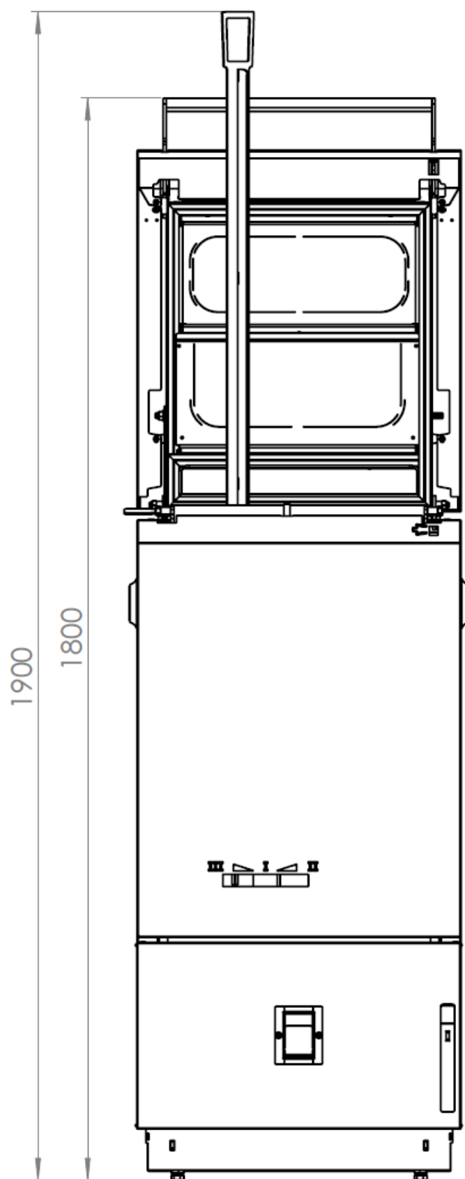
Čelní pohled na kotel s otevřenými horními dvířky + minimální rozměr pro vytažení turbulátorů z kotle BLAZE PRAKTIK COMBI 25 a 40.
