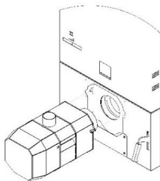
Instalace peletového hořáku do dvírek kotle
