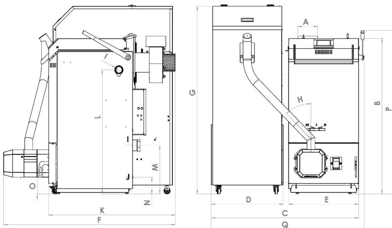
Tabulka 4. Tabulka základních rozměrů kotle BLAZE PRAKTIK COMBI
