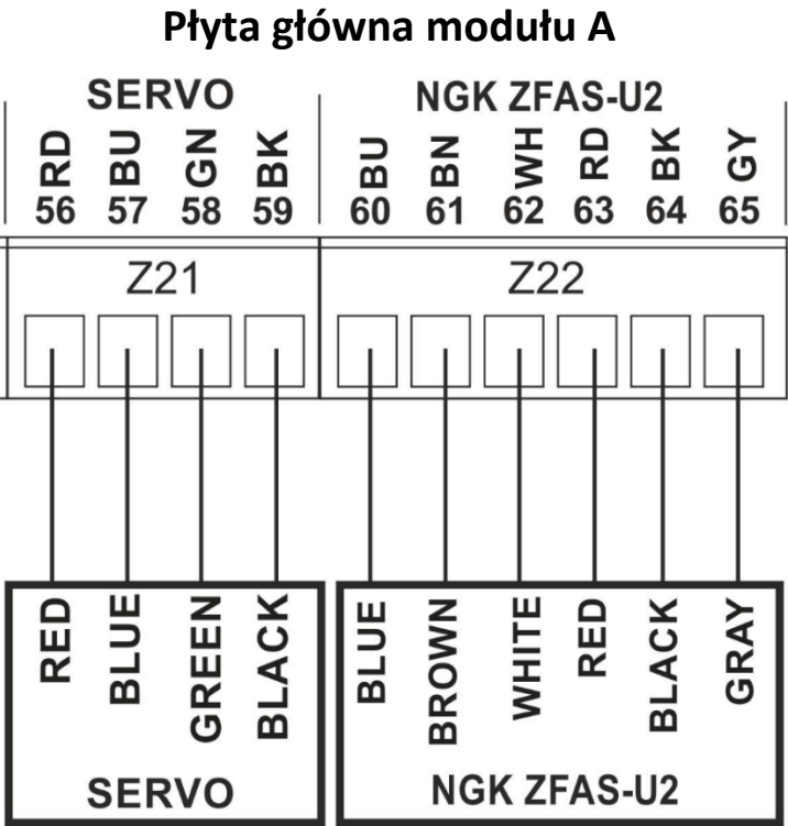
Rysunek 17. Schemat połączeń sondy lambda (NGK ZFAS-U2) i silnika krokowego (SERVO)
