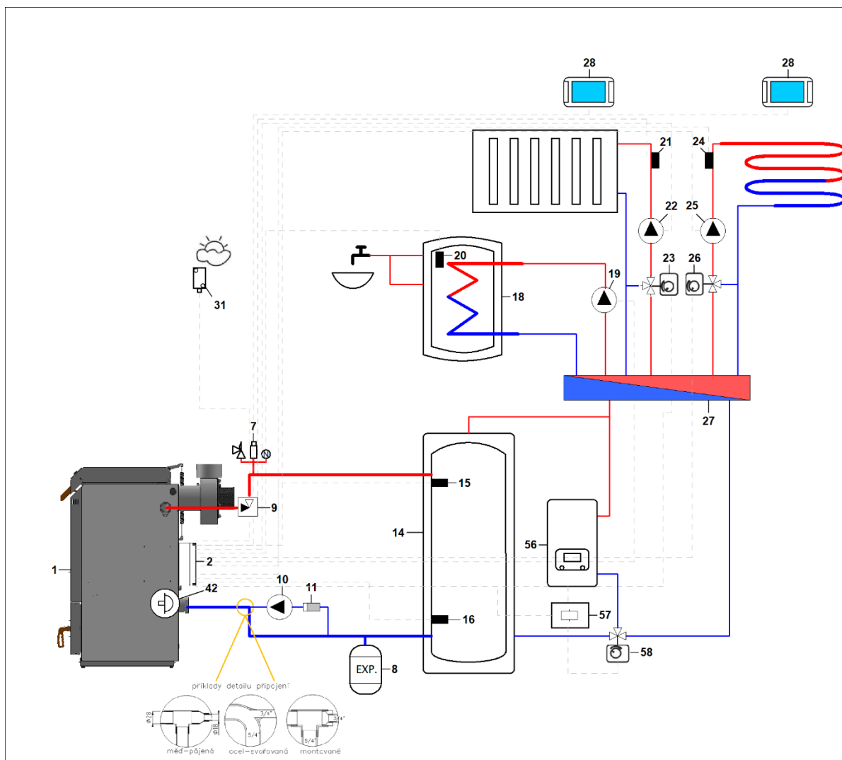
Rysunek 32. Przyłącze hydrauliczne z kotłem rezerwowym (56), przekaźnikiem (57) i zaworem przełączającym (58)
