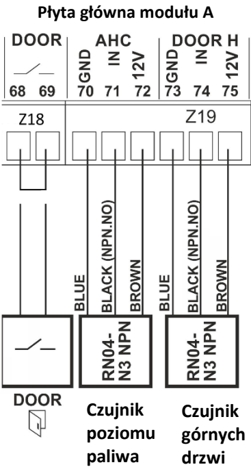
Rysunek 18. Schemat elektryczny czujników indukcyjnych
