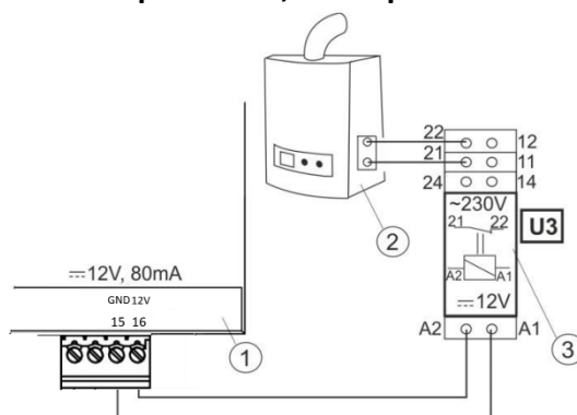
Figura 27. Collegamento elettrico della caldaia di riserva:
