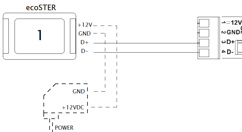
Figura 25. Collegamento a due conduttori del pannello ambiente ecoSTER
