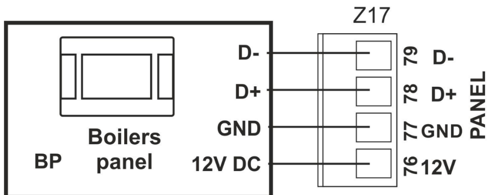
Figura 13. Schema elettrico di collegamento del pannello di controllo del regolatore
