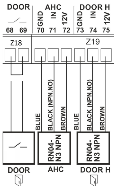
Figura 16. Schema elettrico di collegamento dei sensori induttivi
