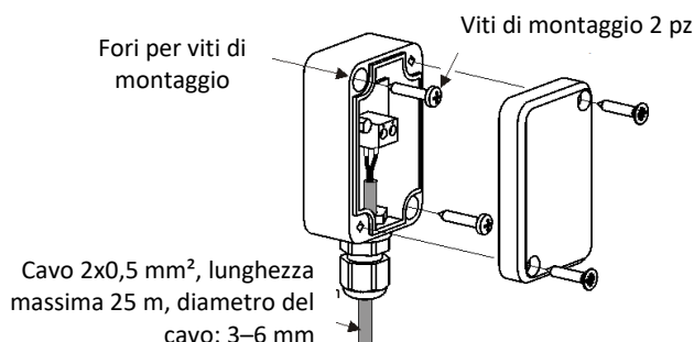
Figura 19. Collegamento della sonda di temperatura esterna CT10P (non inclusa nella dotazione standard della caldaia)
