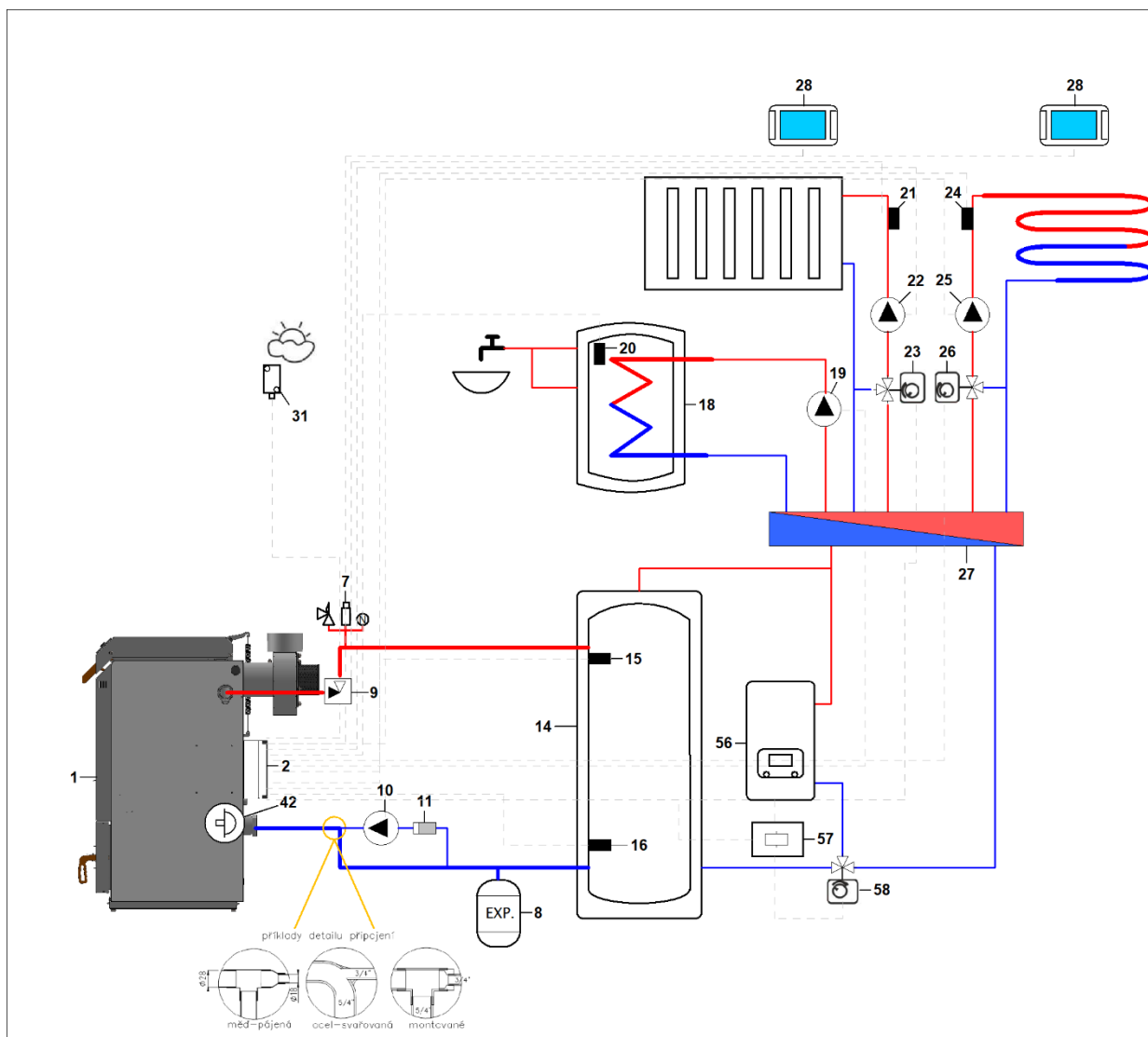
Figura 29: Collegamento idraulico con caldaia di riserva (56) e valvola deviatrice (58)
