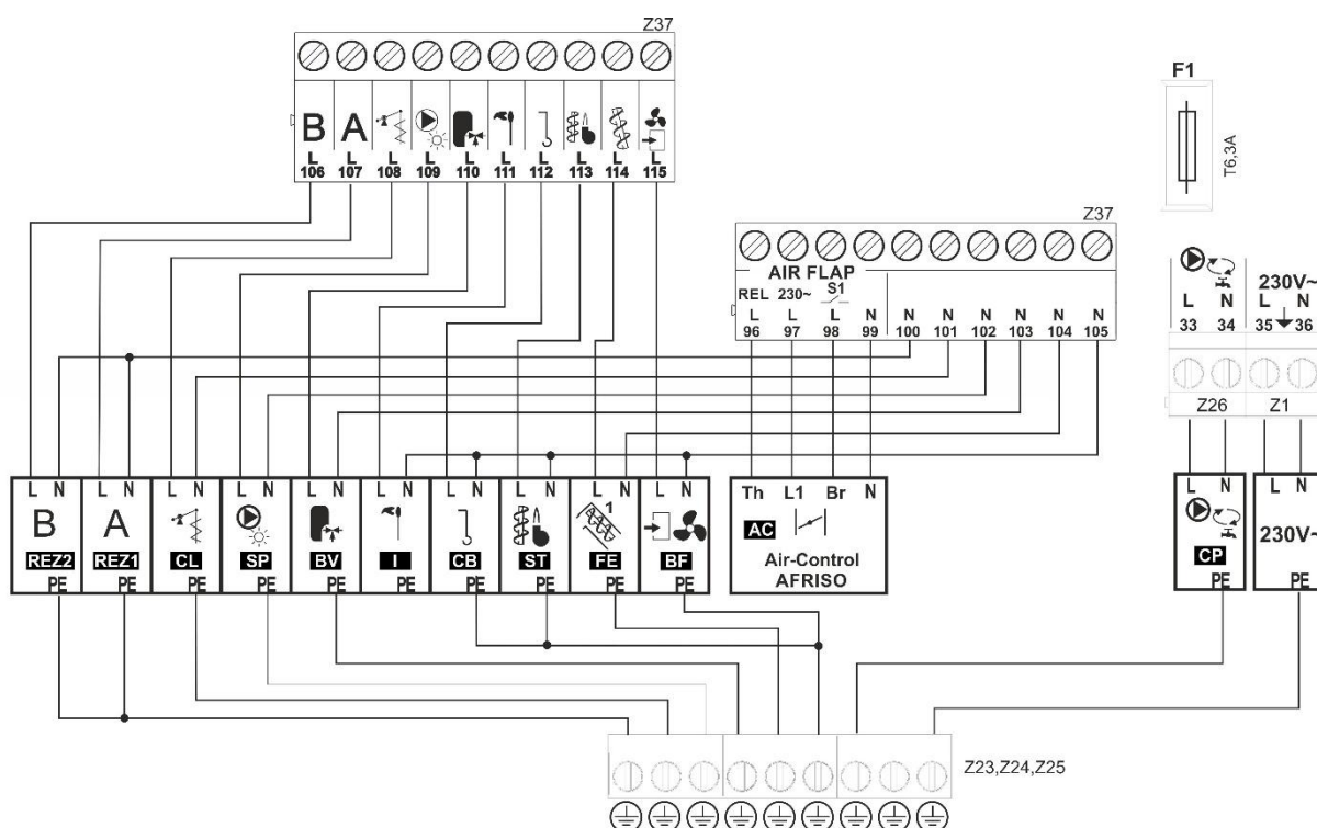
Figura 31. Collegamento di altre periferiche 1
