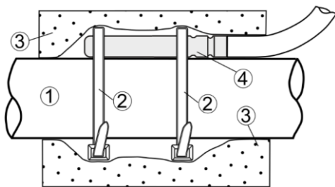
Figura 17. Installazione della sonda di temperatura sul tubo, dove è: 1 - tubo, 2 - fascetta, 3 - isolamento termico, 4 - sonda di temperatura
