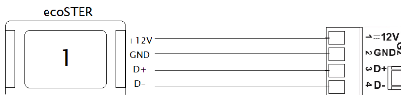
Figura 24. Collegamento a quattro conduttori del pannello ambiente ecoSTER
