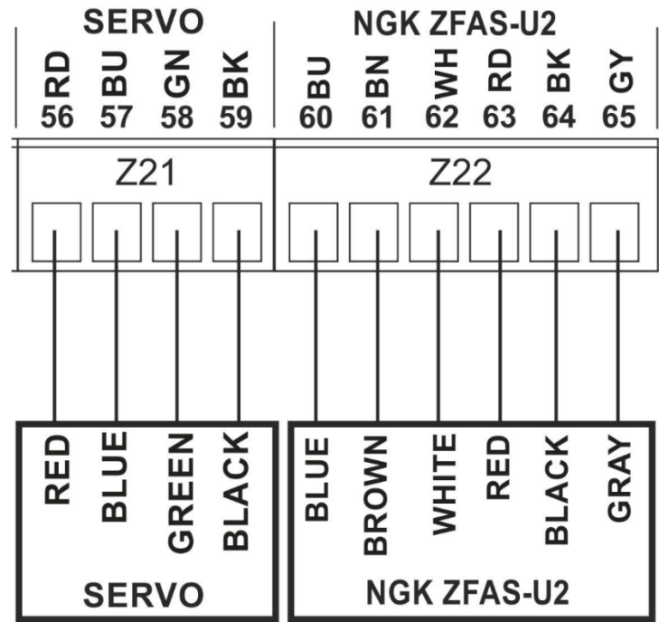
Figura 15. Schema elettrico di collegamento della sonda lambda (NGK ZFAS-U2) e del motore passo-passo (SERVO)
