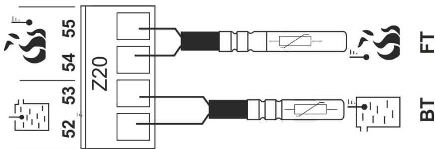
Figura 18. Collegamento delle sonde di temperatura,
