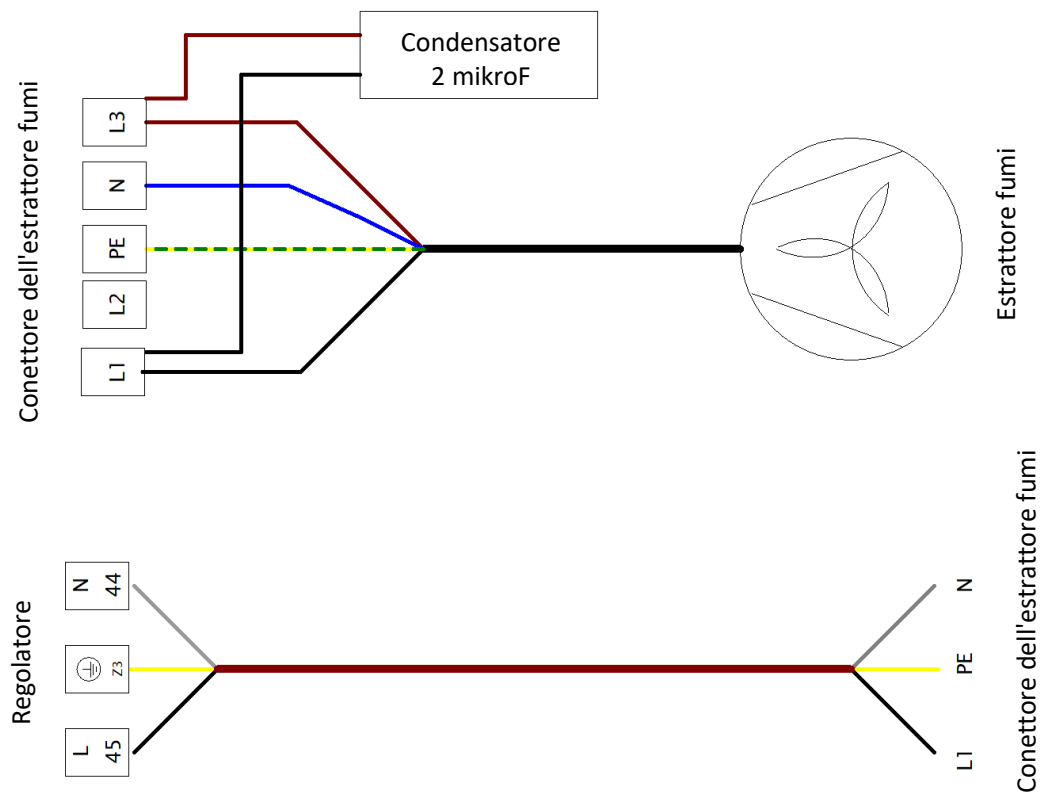
Figura 14. Schema elettrico di collegamento dell'estrattore fumi
