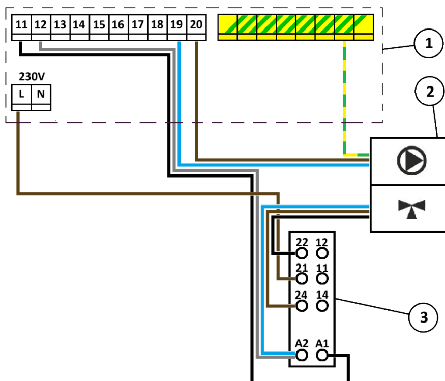
Obrázek 21. Připojení čerpadlové skupiny, kde: 1- regulátor, 2 – čerpadlová skupina, 3 - relé
