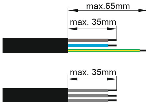
Obrázok 11. Dĺžka odizolovania kábla
