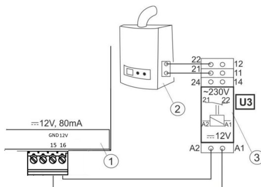
Obrázok 27. Elektrické pripojenie záložného kotla:
