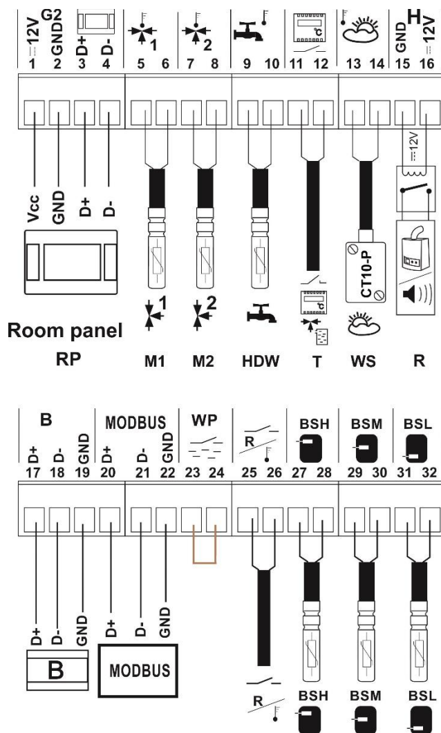
Obrázok 20. Elektrická schéma pripojenia senzora a izbového panela
