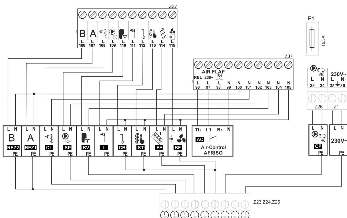
Obrázok 31. Pripojenie ďalších periférnych zariadení 1
