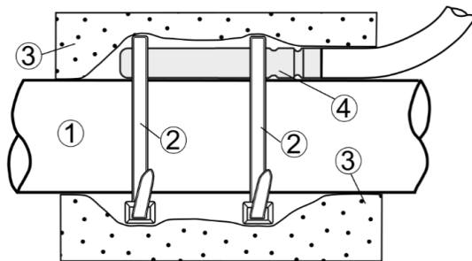
Obrázok 17. Inštalácia teplotného senzora na potrubí,
