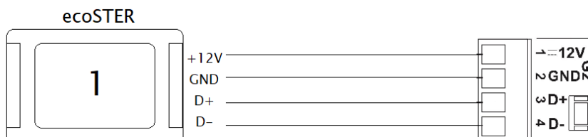
Obrázok 24. Štvorvodičové pripojenie izbového panela ecoSTER
