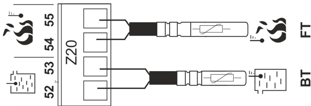
Obrázok 18. Pripojenie teplotných senzorov,
