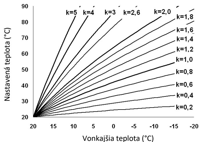
Obrázok 6. Ekvitermálne krivky
