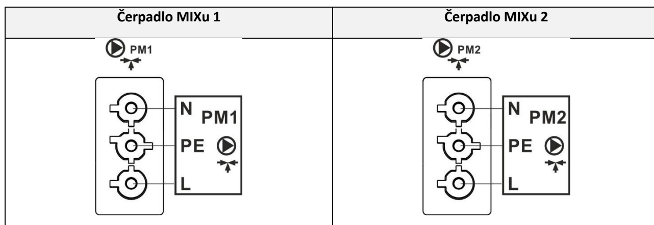
Obrázok 22. Schéma elektrického zapojenia čerpadiel MIXu
