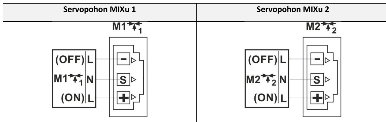
Obrázok 23. Schéma elektrického zapojenia servopohonov MIXu
