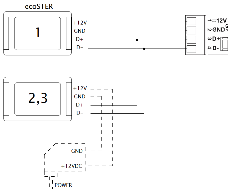
Obrázok 26. Kombinované pripojenie izbového panela ecoSTER
