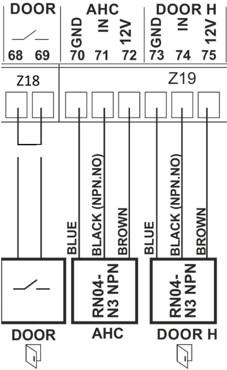
Obrázok 16. Schéma elektrického zapojenia indukčných senzorov
