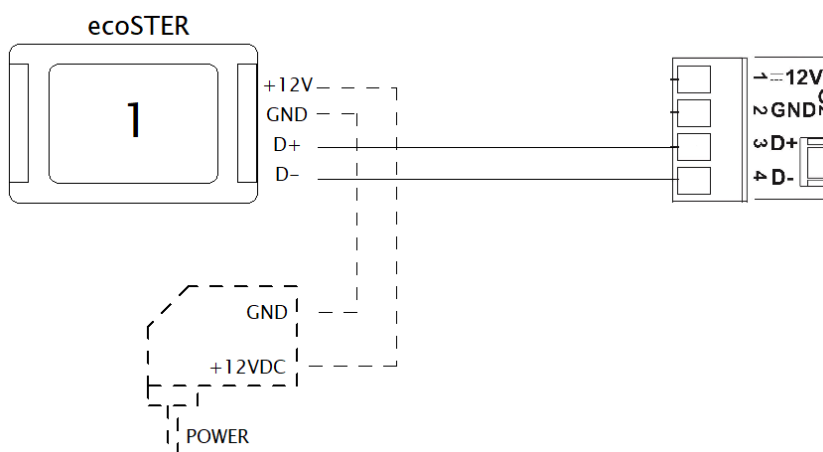
Obrázok 25. Dvojvodičové pripojenie izbového panela ecoSTER
