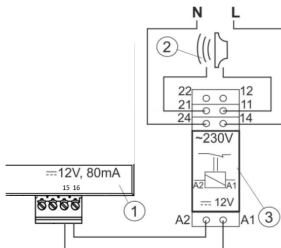
Obrázok 30. Pripojenie externého zariadenia na signalizáciu alarmu, kde: 1 – regulátor, 2 – externé zariadenie na signalizáciu alarmu, 3 – relé
