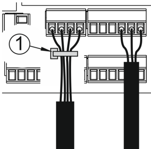
Obrázok 12. Dĺžka odizolovania kábla, kde: 1 – káblová spona
