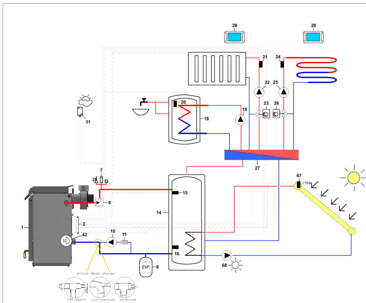
Obrázok 8. Hydraulické pripojenie so solárnym kolektorom:
