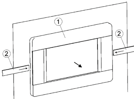
Obrázok 10. Demontáž ovládacieho panela
