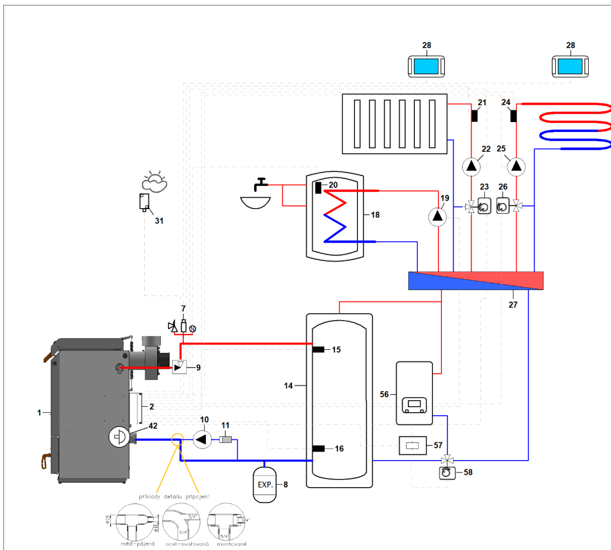
Obrázok 29. Hydraulické pripojenie so záložným kotlom (56) a prepínacím ventilom (58)
