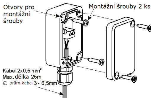
Obrázok 19. Pripojenie vonkajšieho teplotného senzora CT10P (nie je súčasťou základnej výbavy kotla)
