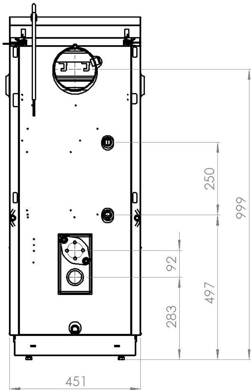
Zadní pohled na kotel BLAZE GREEN 10 s rozměry
