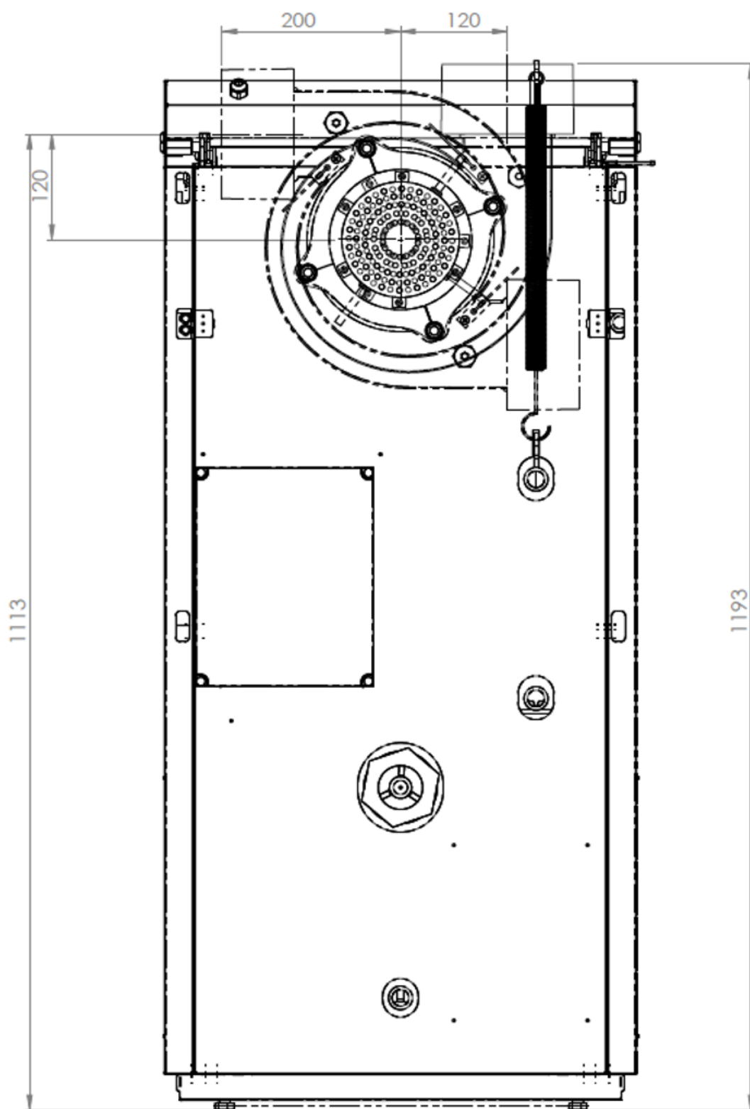
Zadní pohled na kotel BLAZE GREEN 18, 26 a 33 s rozměry
