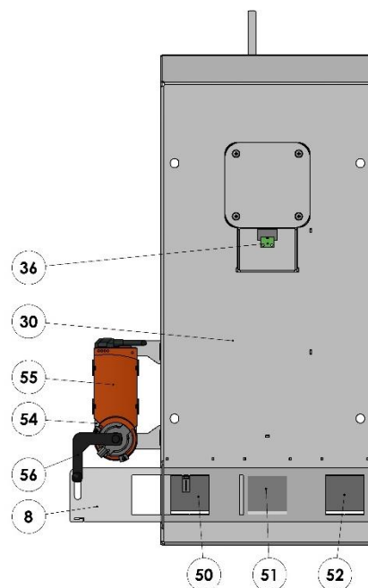
Schéma kotle – detail vzduchování
