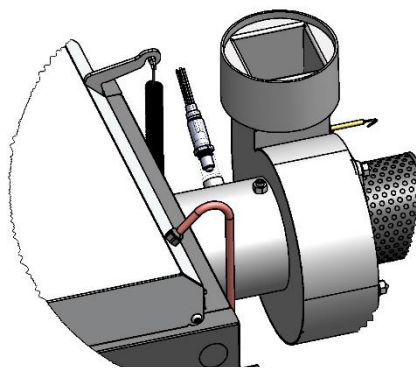
Instalace lambda sondy
