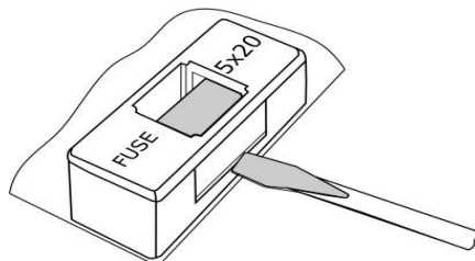
Obrázek 8. Výměna síťové pojistky
