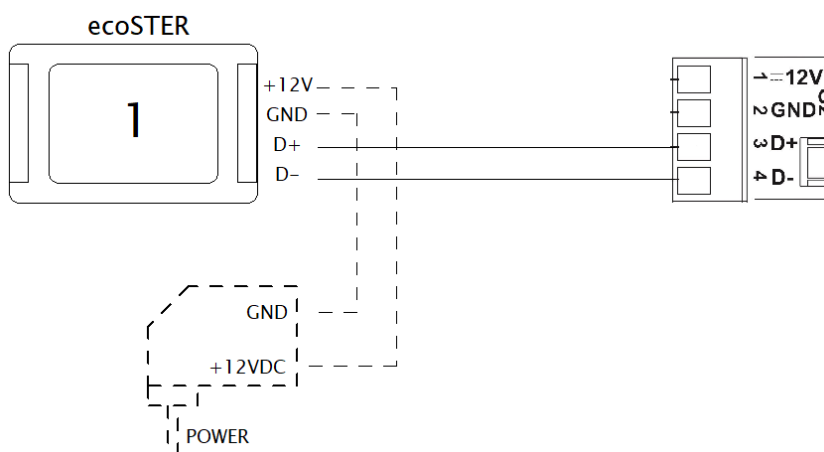
Obrázek 24. Dvouvodičové připojení pokojového panelu ecoSTER
