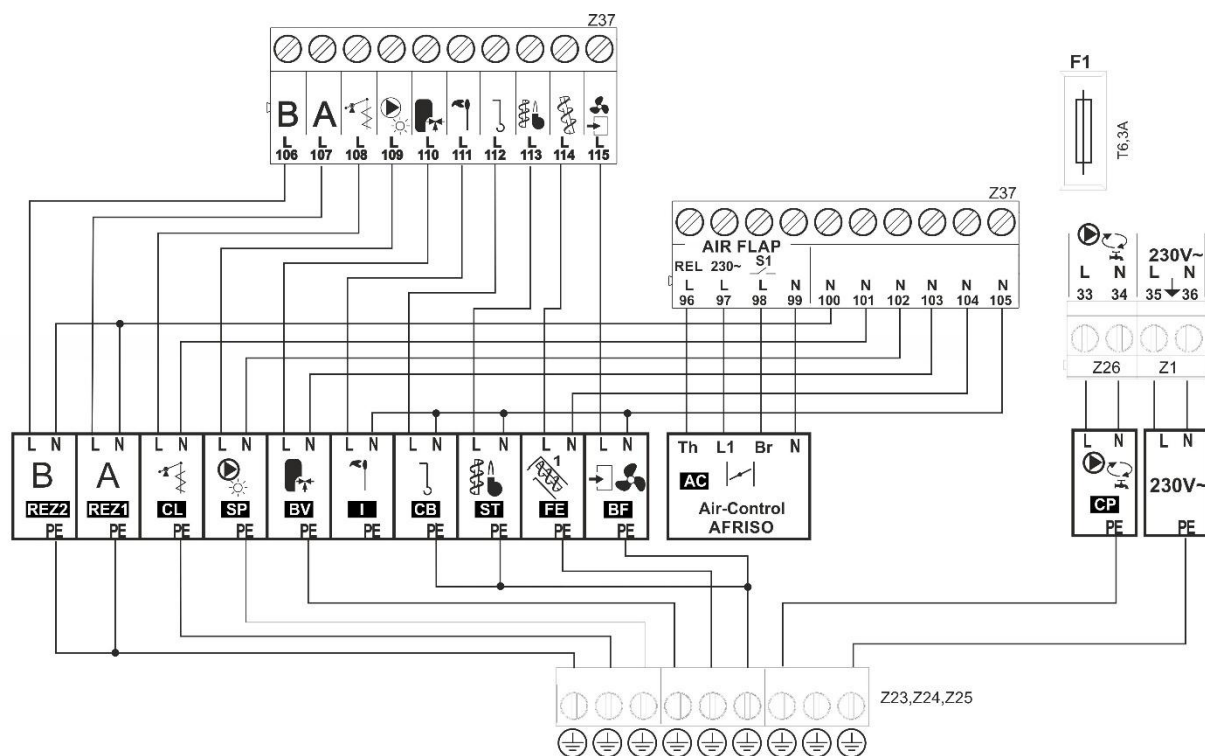
Obrázek 30. Připojení ostatních periférií 1
